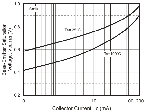
Fig.3 - V_{BE(sat)} - I_c
