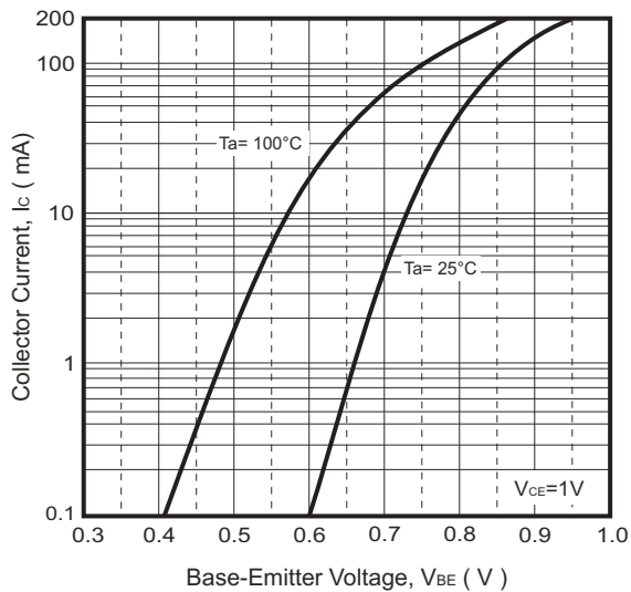
Fig.5 - I_c - V_{BE}
