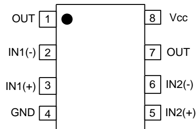
SOP-8 / TSSOP-8
