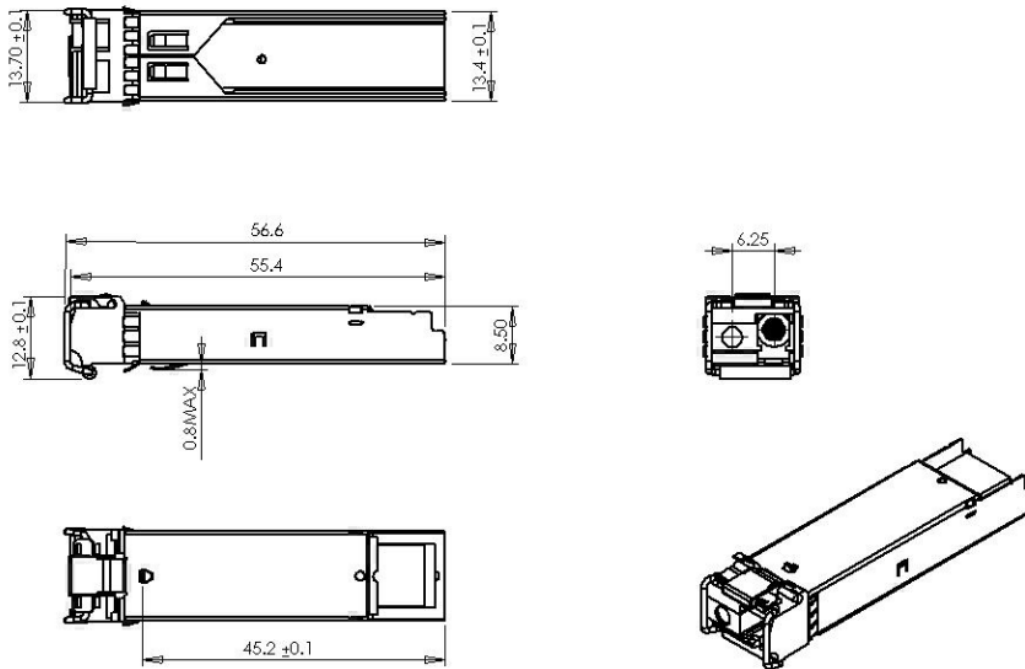
MSFP-155M-BIDI40
