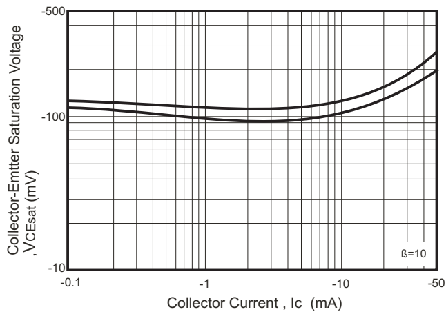
Fig.3 - V_{CEsat} - I_c
