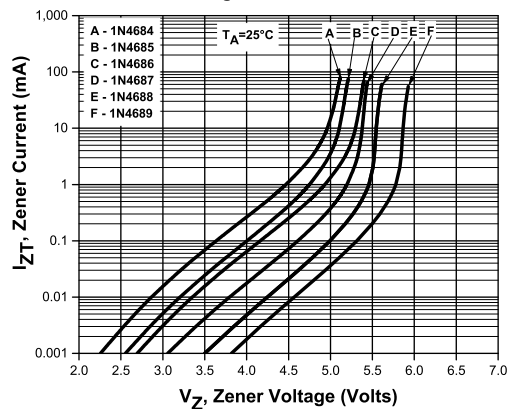
Zener Voltage, 1N4684-1N4689
