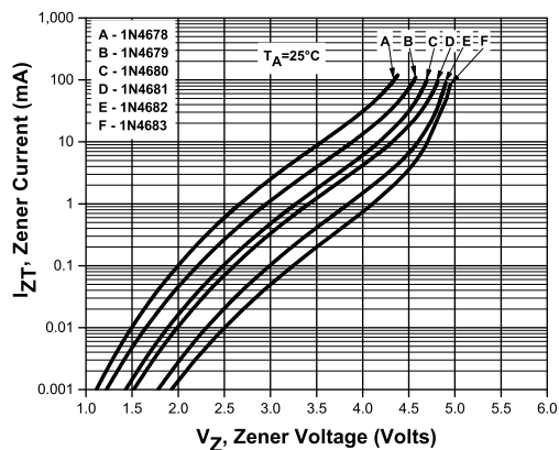
Zener Voltage, 1N4678-1N4683
