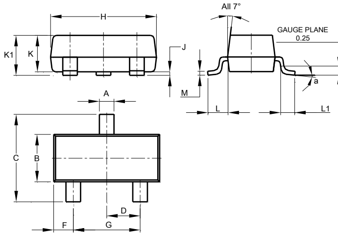
SOT23
