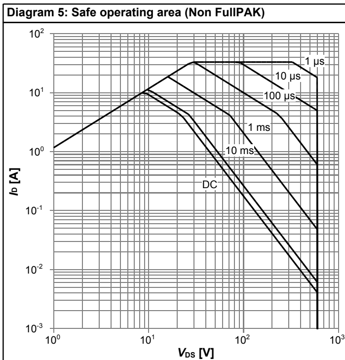
I_D=f(V_{DS}); T_C=25\text{ °C}; D=0; \text{parameter: } t_p
