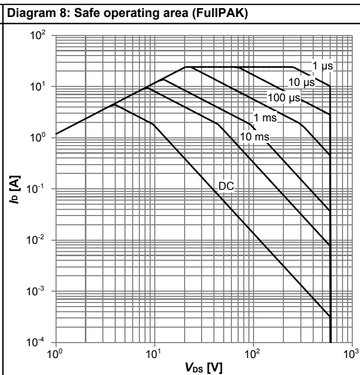
I_D=f(V_{DS}); T_C=80\text{ °C}; D=0; \text{parameter: } t_p
