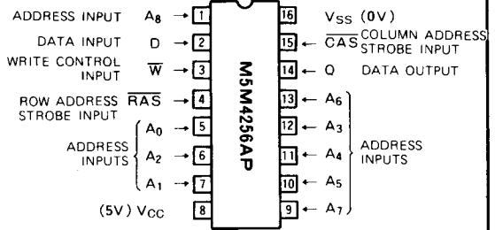
Outline 16P4H(DIP)
