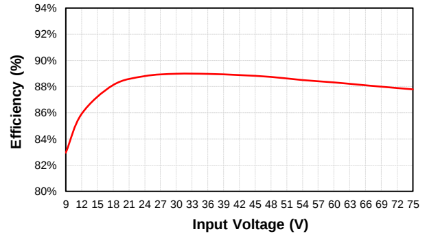
CQB100W8-36S12 Eff Vs Vin @25 Deg. C
