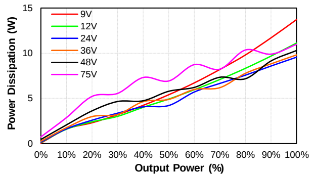
CQB100W8-36S28 Pd Vs Po @25 Deg. C
