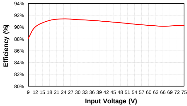
CQB100W8-36S28 Eff Vs Vin @25 Deg. C
