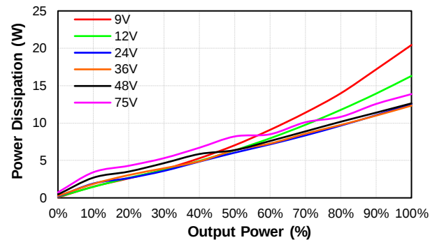
CQB100W8-36S12 Pd Vs Po @25 Deg. C
