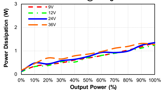
EC2SBW-24D15H Pd Vs Po @25 Deg. C
